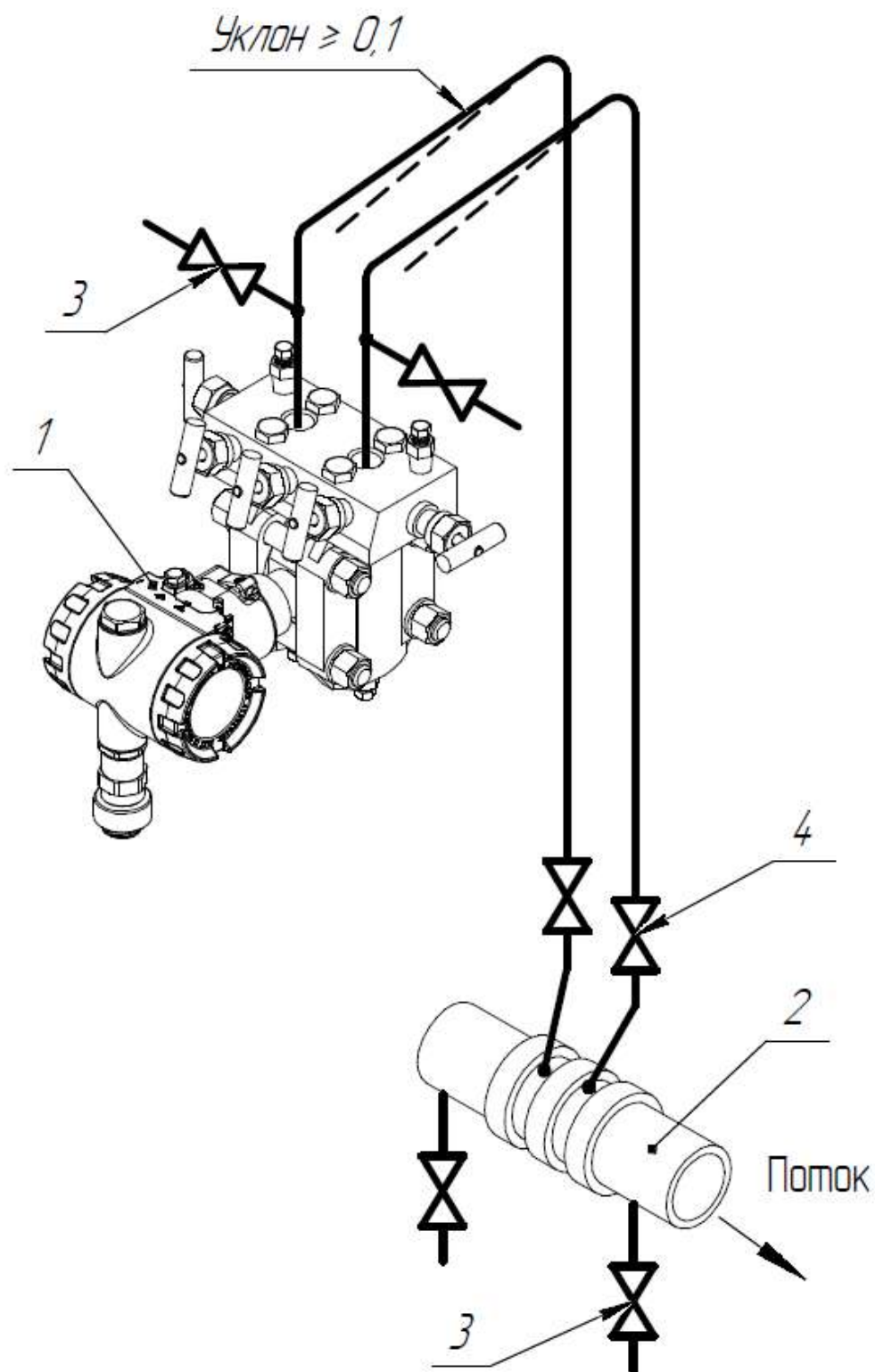
Рисунок Д.2.7 – Подключение СДВ-SMART для измерения расхода газа выше сужающего устройства:
