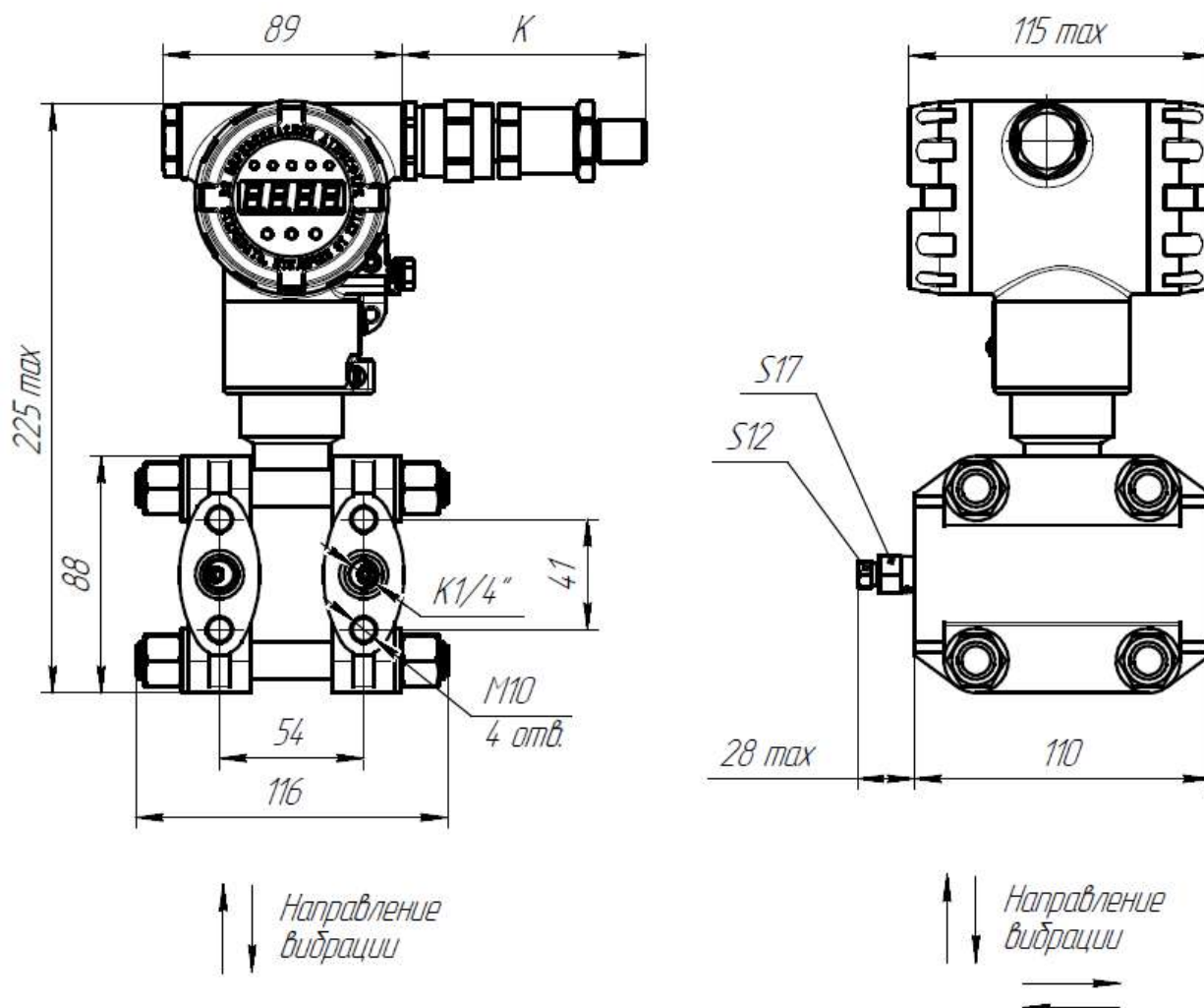
Рисунок Б.2 – Габаритный чертеж преобразователей избыточного давления, разрезения, давления-разрезения, разности давлений с конструктивным исполнением S, Op-S, Астр-S, М-S по таблице А.5
