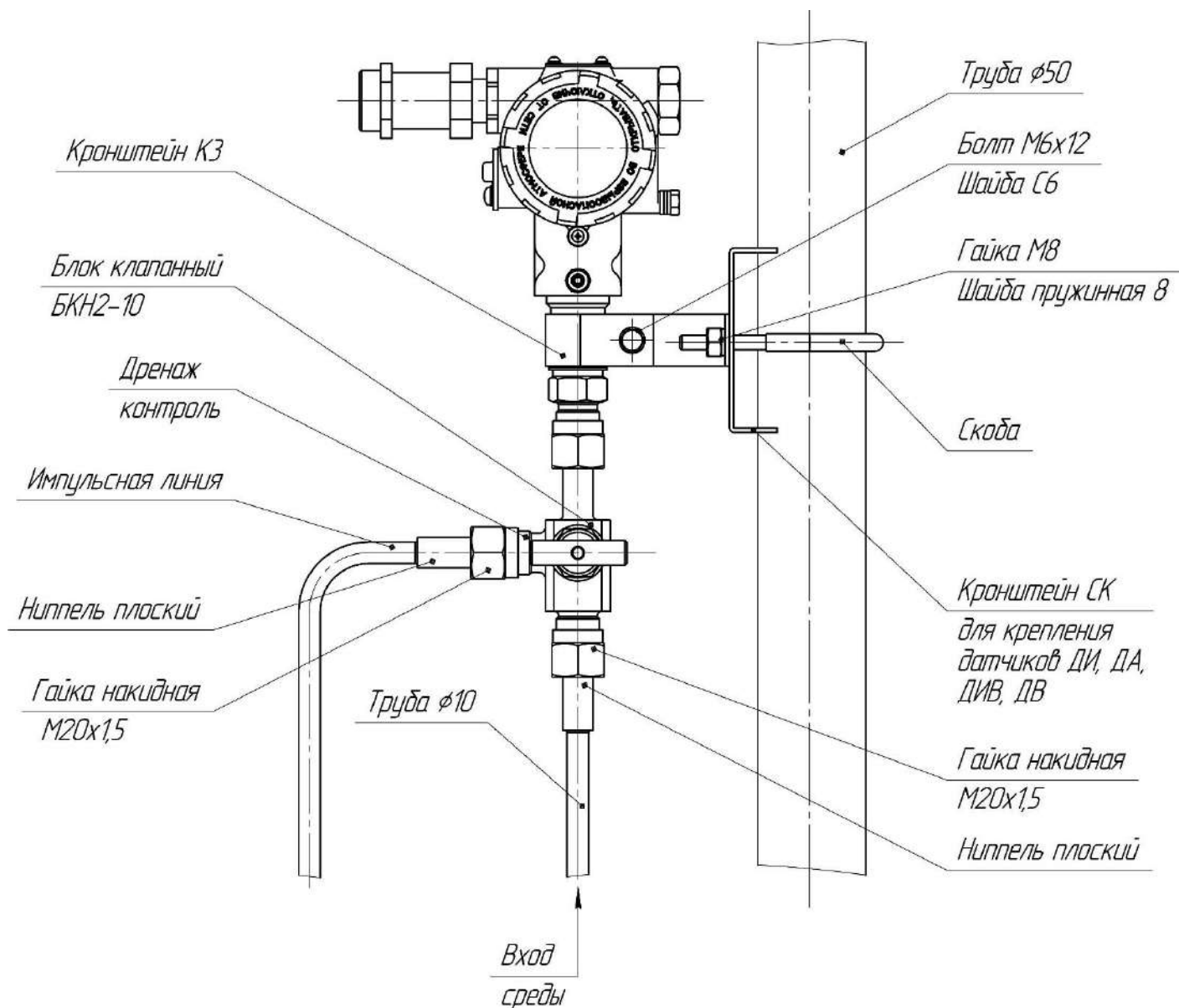
Рисунок Д.1 – Монтажный чертеж установки преобразователя давления штуцерного конструктивного исполнения с монтированным клапанным блоком «БКН» резьбового присоединения к импульсным линиям, и с КМЧ «Ниппель М20» и «Кронштейн СК» («Кронштейн КЗ» входит в комплект) для крепления датчиков ДИ, ДА, ДИВ, ДВ
