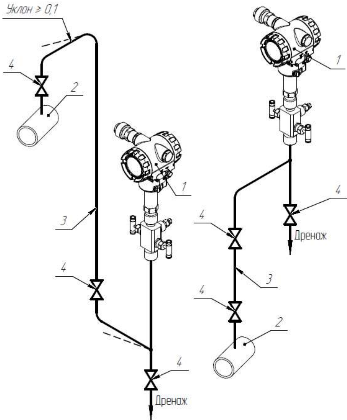
Рисунок Д.1.5 – Подключение СДВ-SMART для измерения давления сухого газа:
