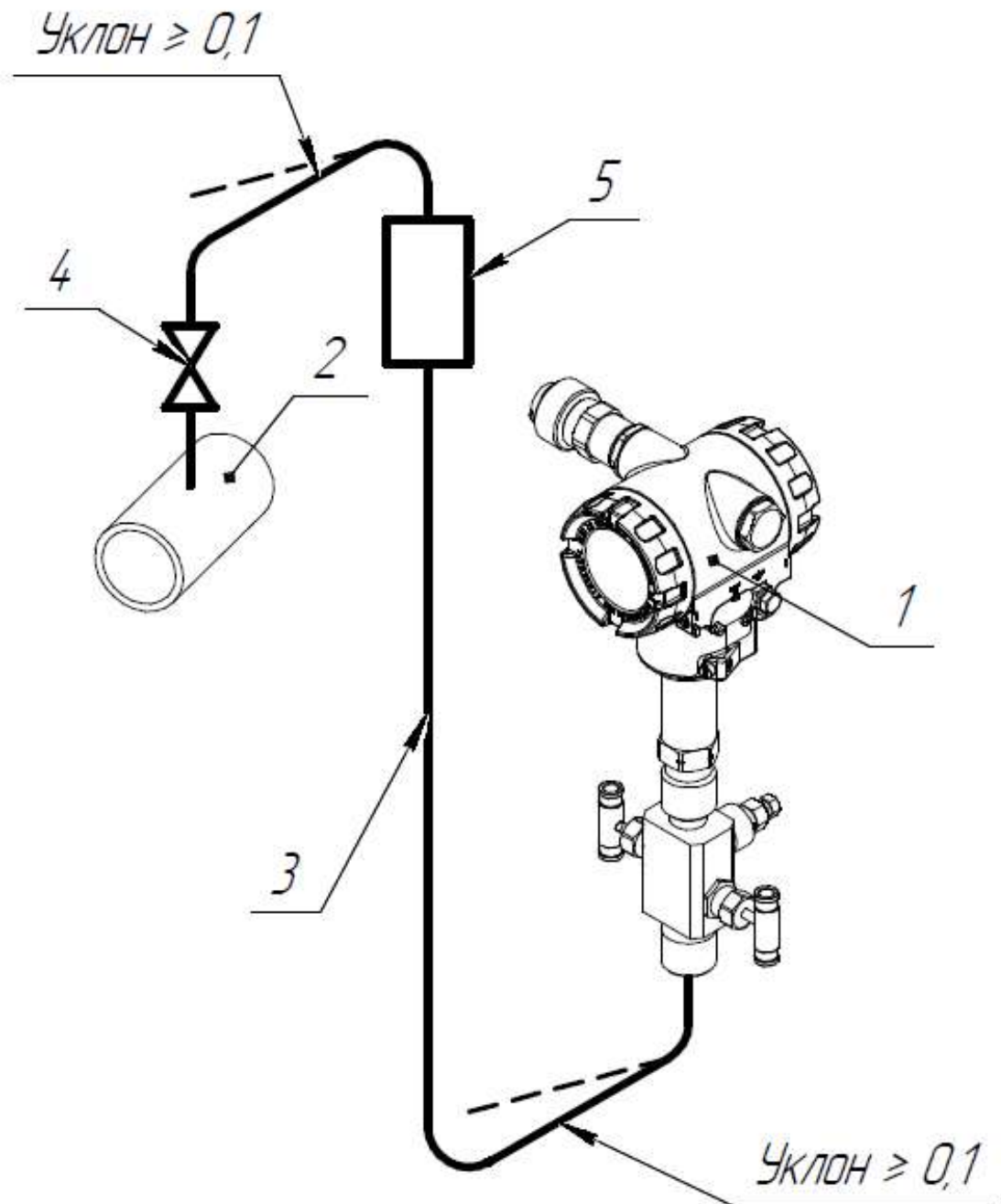
Рисунок Д.1.8 – Подключение СДВ-SMART для измерения давления агрессивного газа выше точки отбора:
