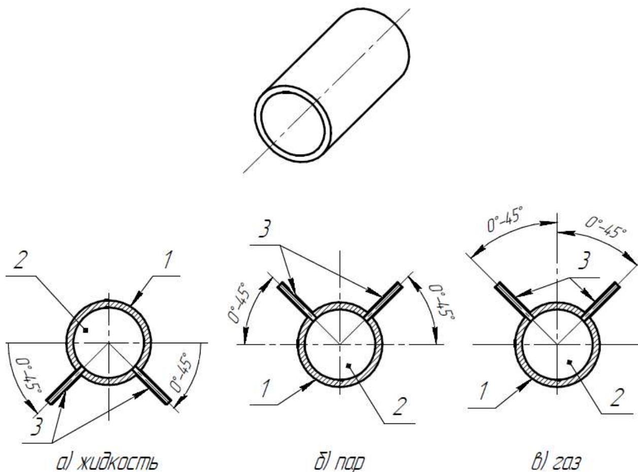
Рисунок Д.1.2 – Подключение импульсной линии к горизонтальному трубопроводу:
