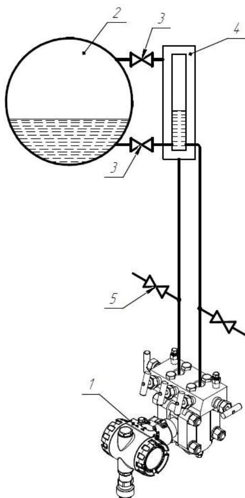
Рисунок Д.2.9 – Подключение СДВ-SMART для измерения уровня жидкости в паровом котле:
