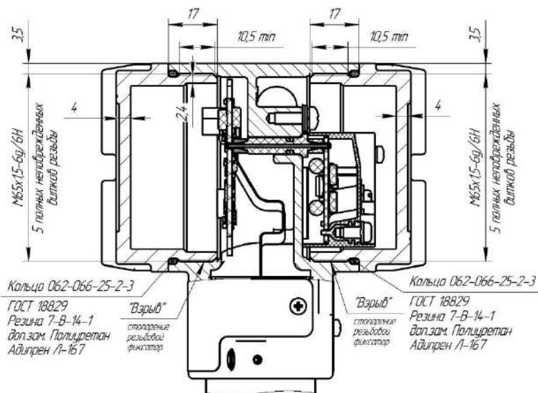
Рисунок Г.4 – Исполнение преобразователя с глухой крышкой
