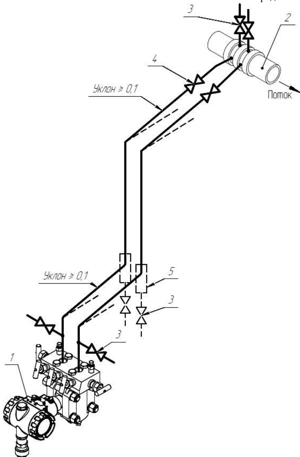
Рисунок Д.2.2 – Подключение СДВ-SMART для измерения расхода жидкости ниже сужающего устройства:
