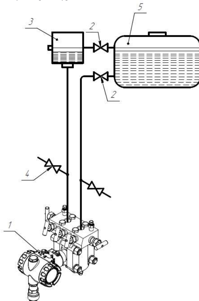
Рисунок Д.2.8 – Подключение СДВ-SMART для измерения уровня жидкости в сосуде под давлением:
