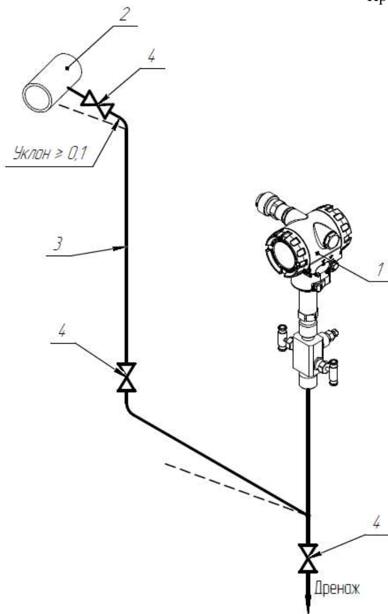
Рисунок Д.1.3 – Подключение СДВ-SMART для измерения давления жидкости или пара ниже точки отбора:
