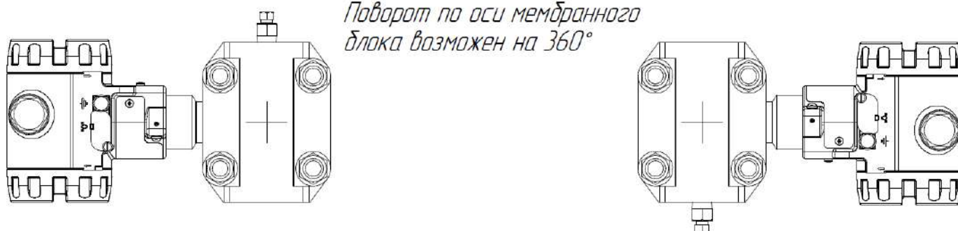
Рисунок Д.4 – Допустимые положения преобразователя давления фланцевого конструктивного исполнения при монтаже (кроме исполнения М-S). Корпус электронного блока преобразователя может быть повернут в любое удобное положение
