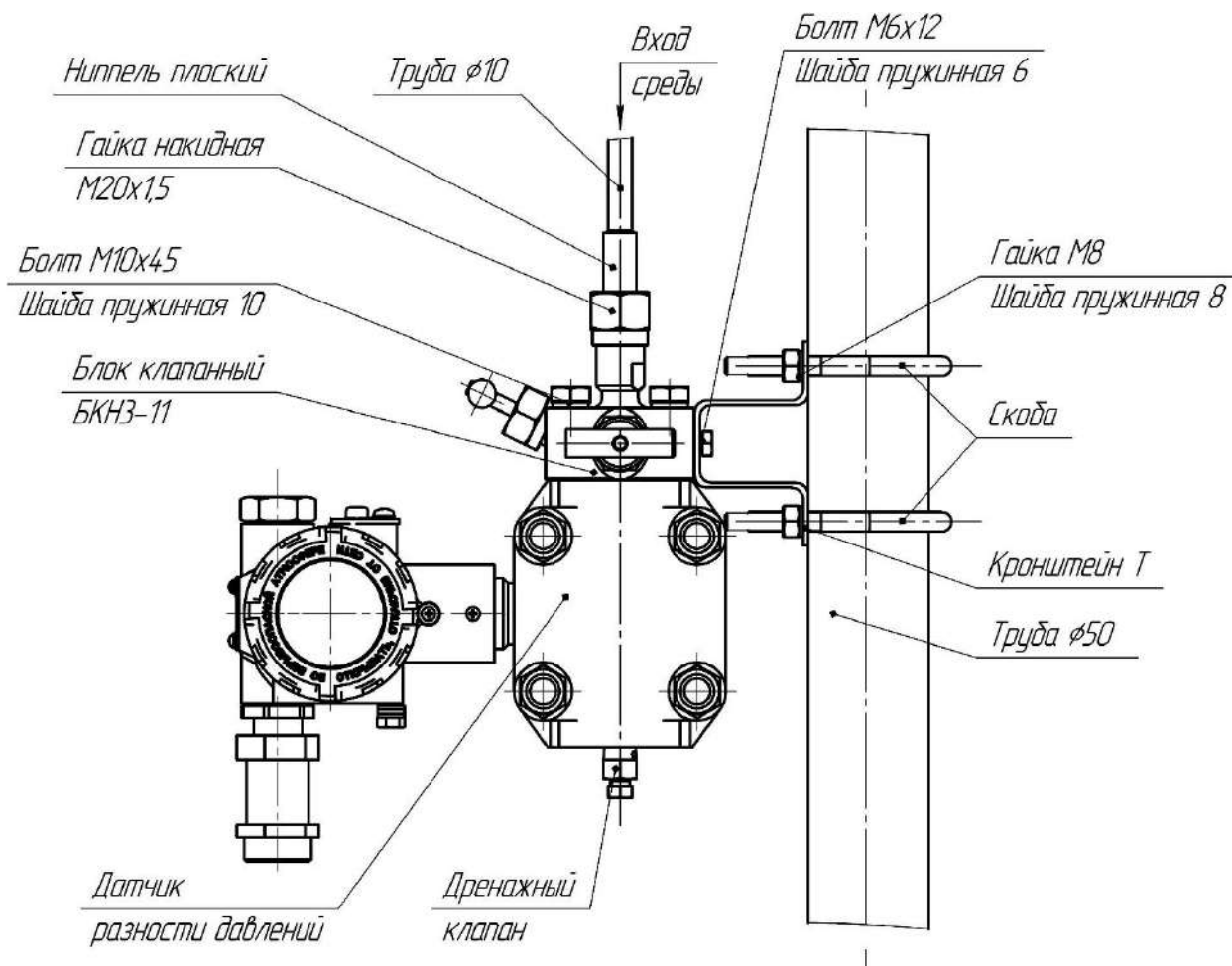
Рисунок Д.3 – Монтажный чертеж установки преобразователя давления фланцевого конструктивного исполнения с монтированным клапанным блоком «БКН» резьбового присоединения к импульсным линиям, и с КМП «Фланец М20» и «Кронштейн Т». Вариант крепления на вертикальной трубе Ø50
