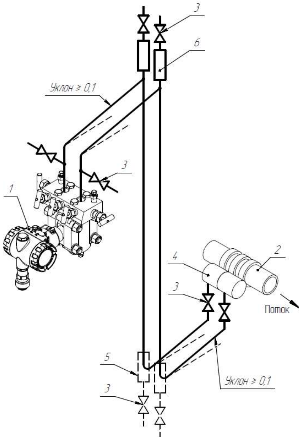
Рисунок Д.2.5 – Подключение СДВ-SMART для измерения расхода пара выше сужающего устройства:
