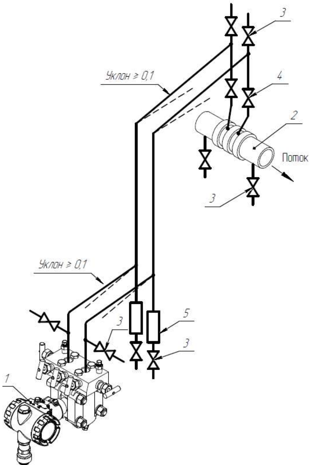
Рисунок Д.2.6 – Подключение СДВ-SMART для измерения расхода газа ниже сужающего устройства:
