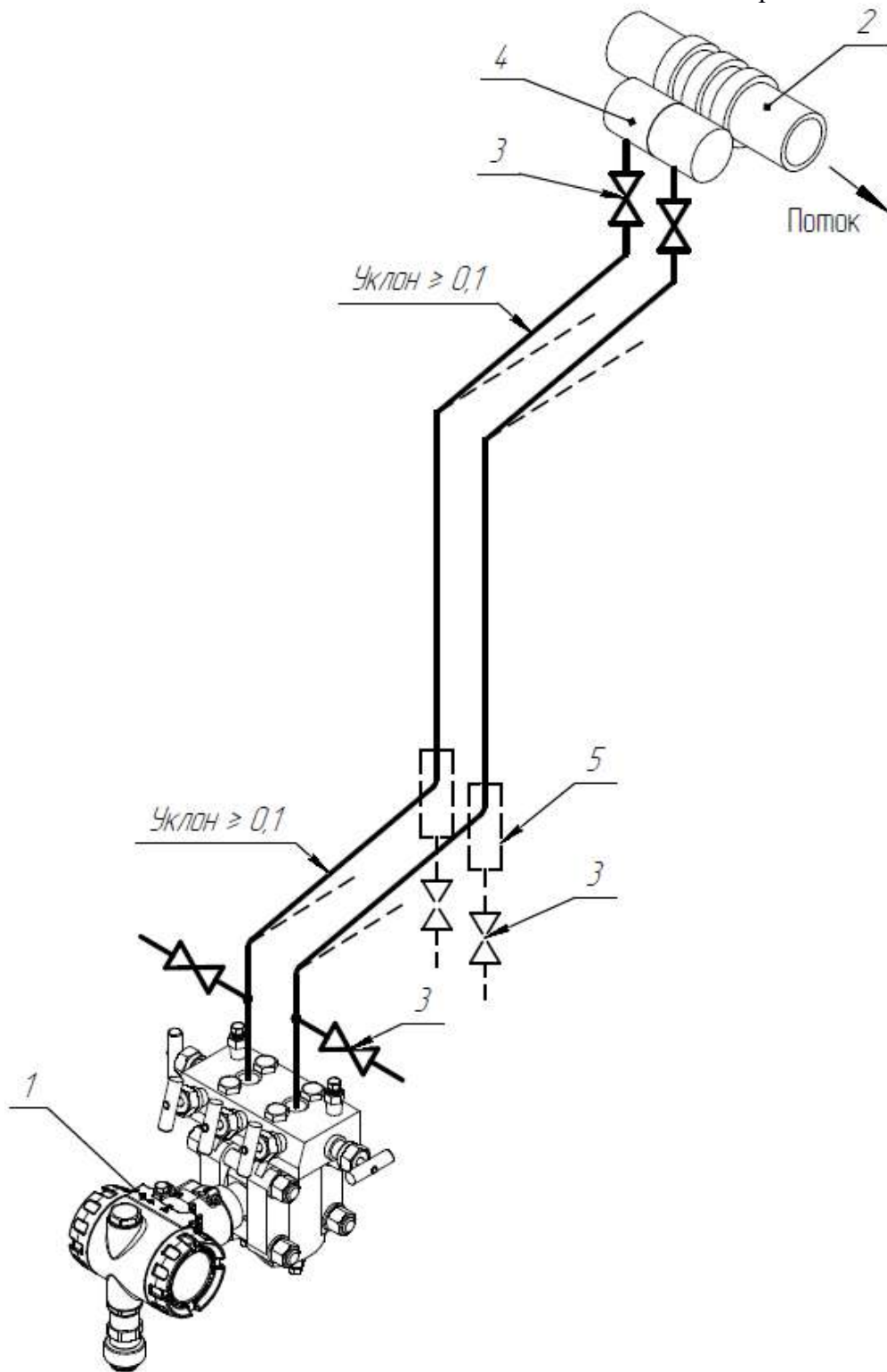
Рисунок Д.2.4 – Подключение СДВ-SMART для измерения расхода пара ниже сужающего устройства:
