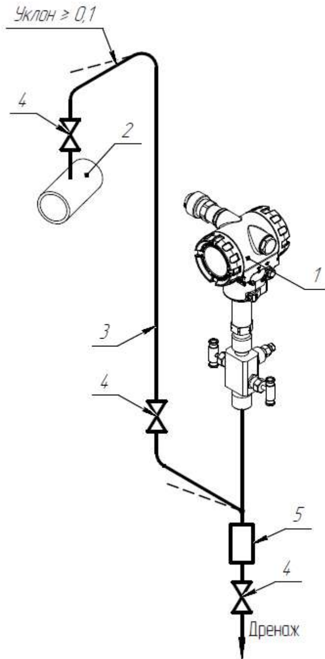
Рисунок Д.1.6 – Подключение СДВ-SMART для измерения давления влажного газа:
