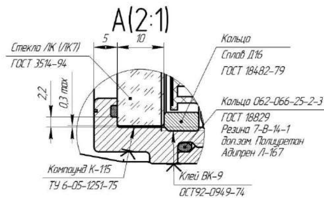
Рисунок Г.2 – Корпус блока электроники
