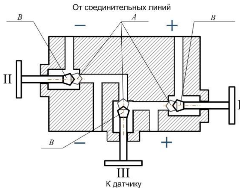
Рисунок 2 — Схема клапанного блока
