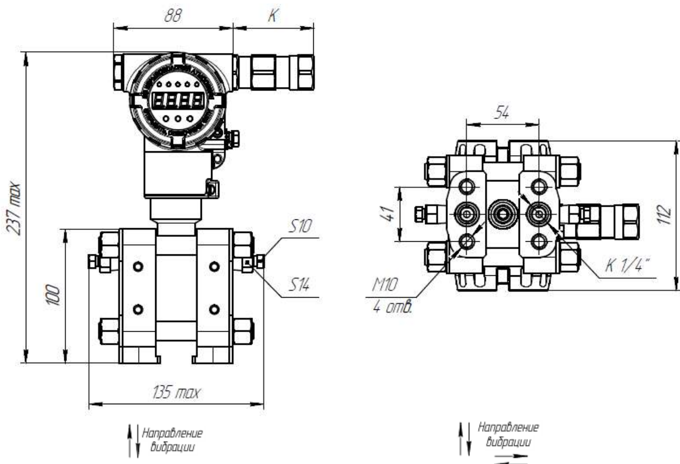
Рисунок Б.3 – Габаритный чертеж преобразователей избыточного давления, разрежения, давления-разрежения, разности давлений с конструктивным исполнением НП-S по таблице А.5
