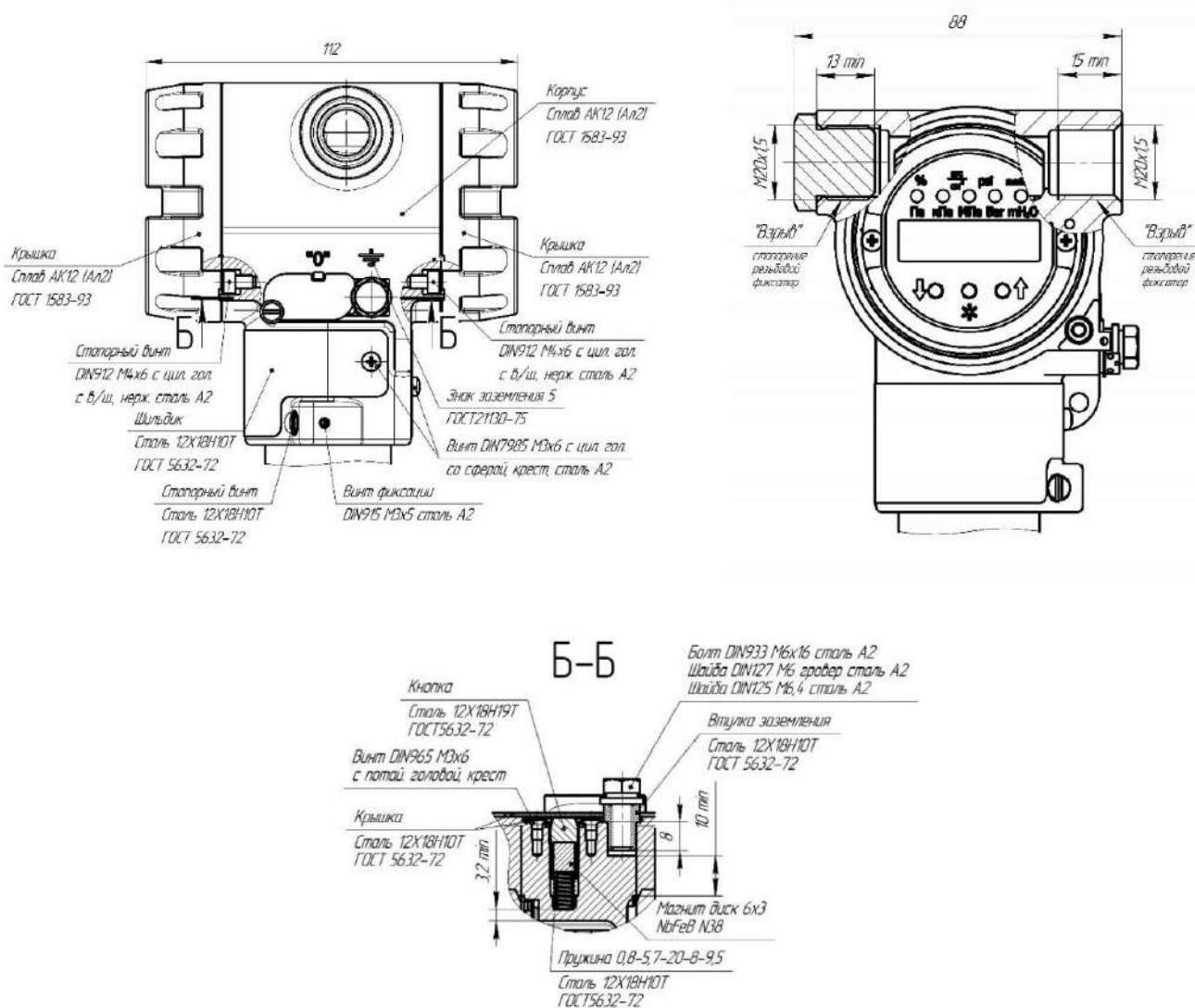
Рисунок Г.1 – Чертеж средств взрывозащиты преобразователей
