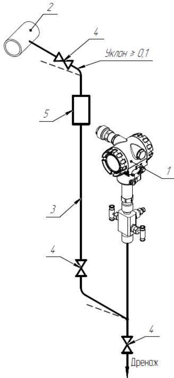
Рисунок Д.1.9 – Подключение СДВ-SMART для измерения давления агрессивной или вязкой жидкости (плотность разделительной жидкости больше плотности измеряемой среды):
