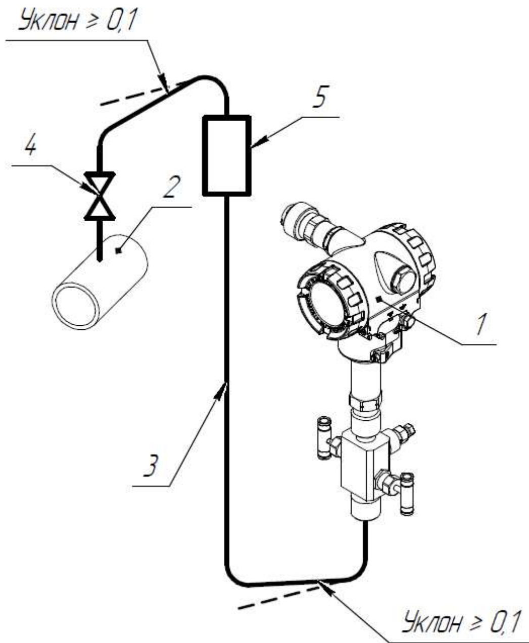
Рисунок Д.1.7 – Подключение СДВ-SMART для измерения давления агрессивного газа ниже точки отбора:
