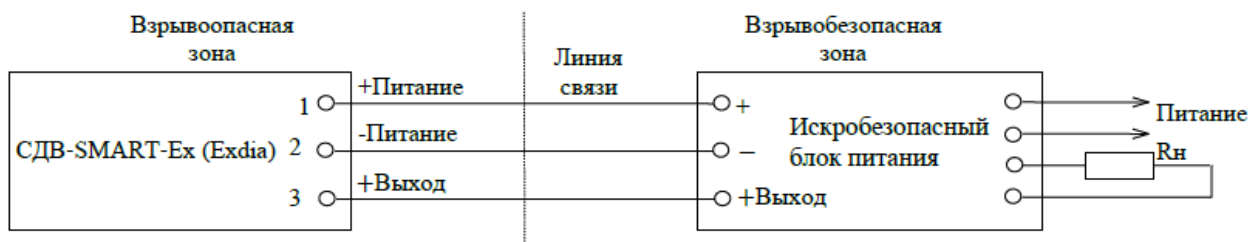
Рисунок В.6 — Схема внешних электрических соединений преобразователей СДВ-SMART-Ex, СДВ-SMART-Exdia
