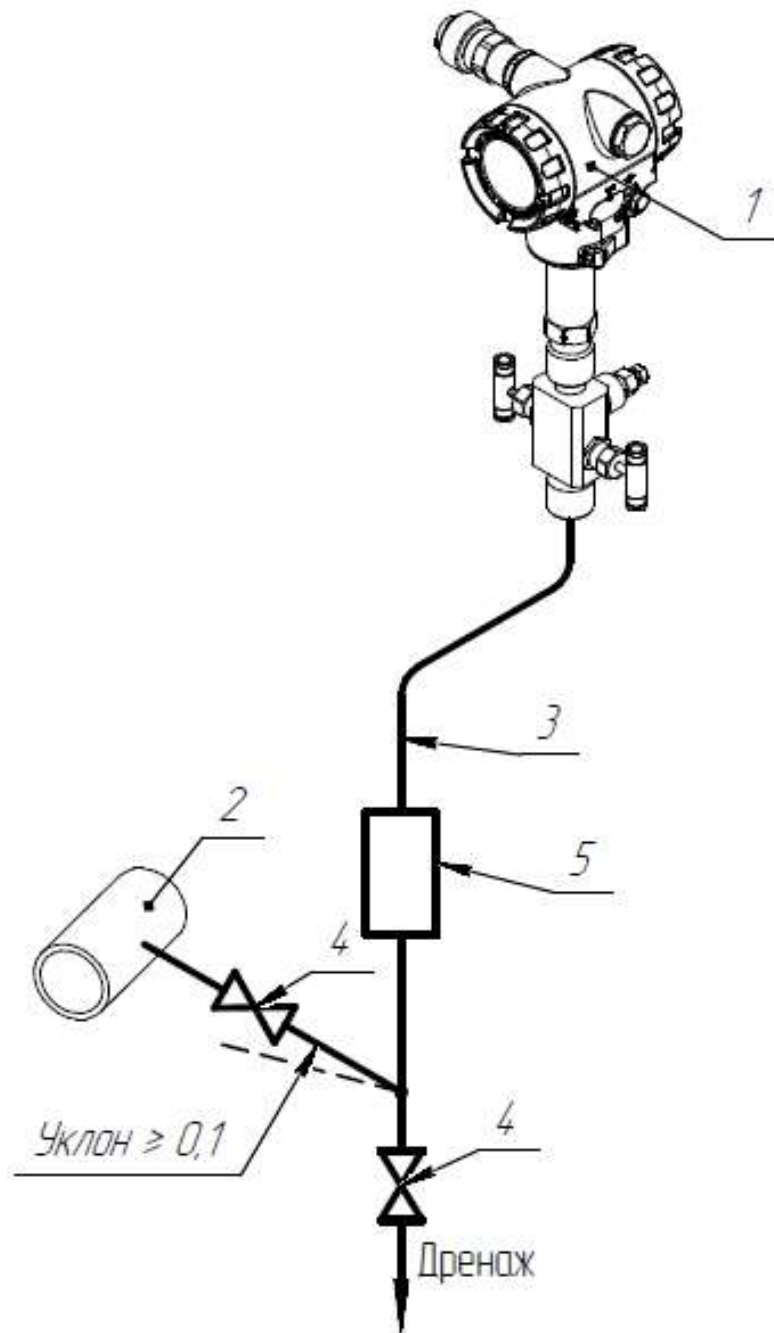
Рисунок Д.1.10 – Подключение СДВ-SMART для измерения давления агрессивной или вязкой жидкости (плотность разделительной жидкости меньше плотности измеряемой среды):
