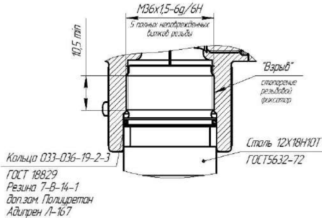
Рисунок Г.5 – Крепление корпуса блока электроники на приемнике давления
