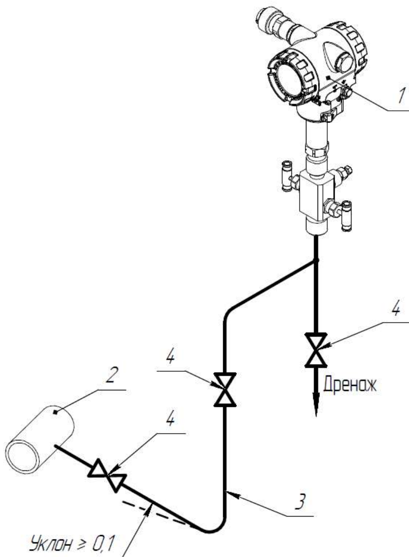
Рисунок Д.1.4 – Подключение СДВ-SMART для измерения давления жидкости или пара выше точки отбора:
