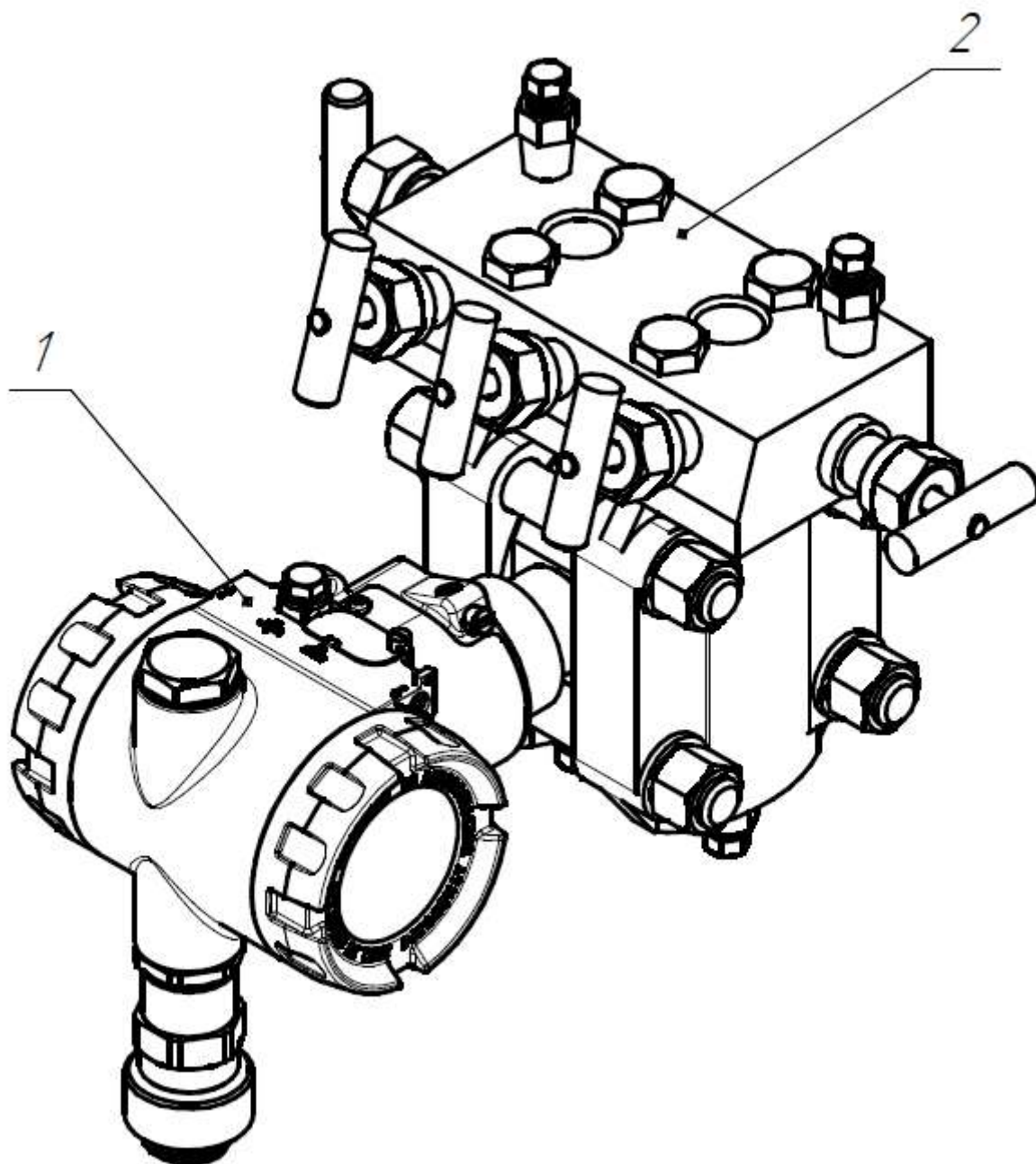
Рисунок Д.2.1 – СДВ-SMART (фланцевое исполнение) (1); Трехвентильный (пятивентильный) клапанный блок (2)
