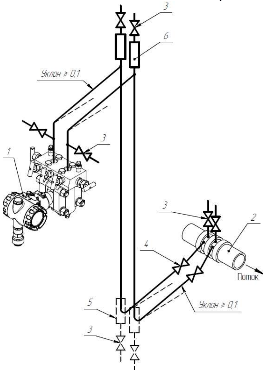
Рисунок Д.2.3 – Подключение СДВ-SMART для измерения расхода жидкости выше сужающего устройства:
