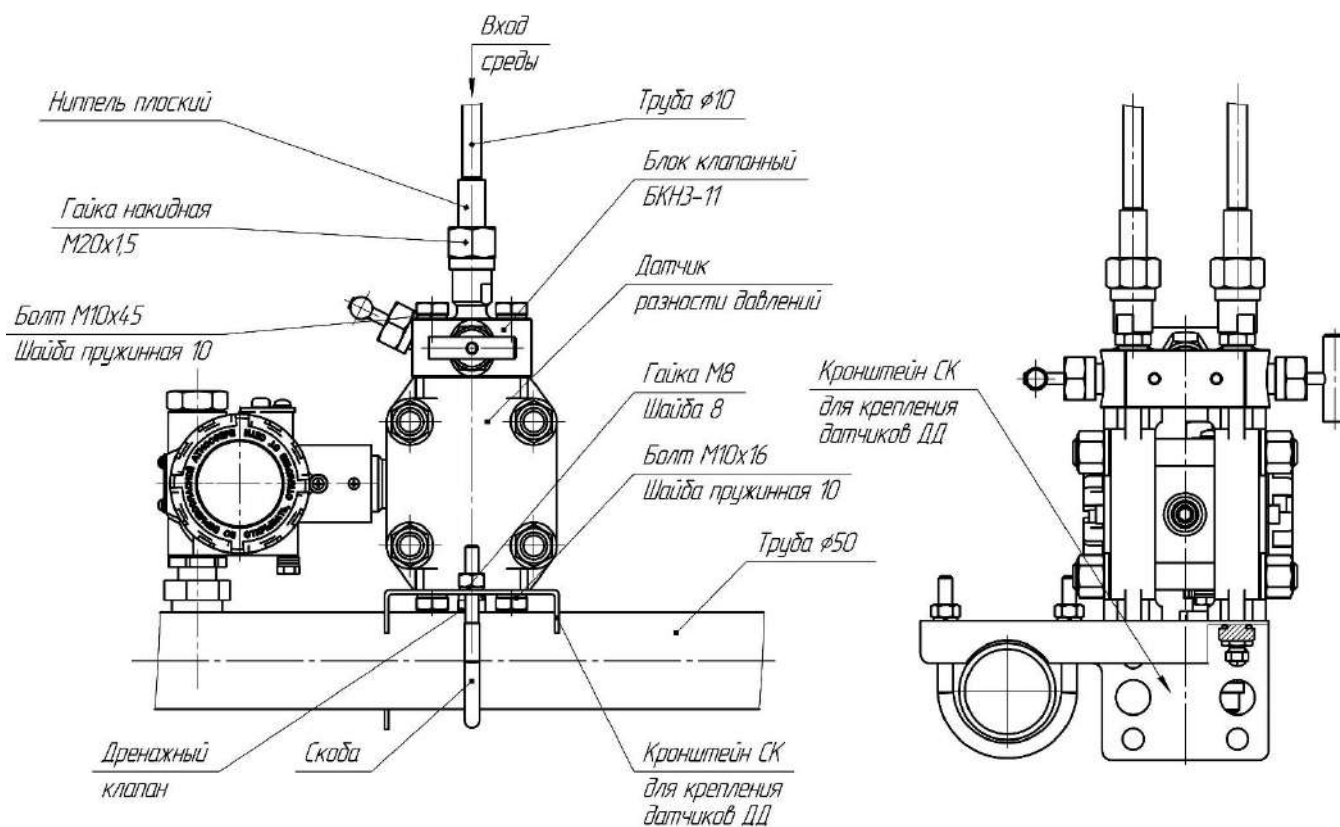
Рисунок Д.2 – Монтажный чертеж установки преобразователя давления фланцевого конструктивного исполнения с монтированным клапанным блоком «БКН» резьбового присоединения к импульсным линиям, и с КМП «Фланец М20» и «Кронштейн СК» (для крепления датчиков ДД). Вариант крепления на горизонтальной трубе Ø50
